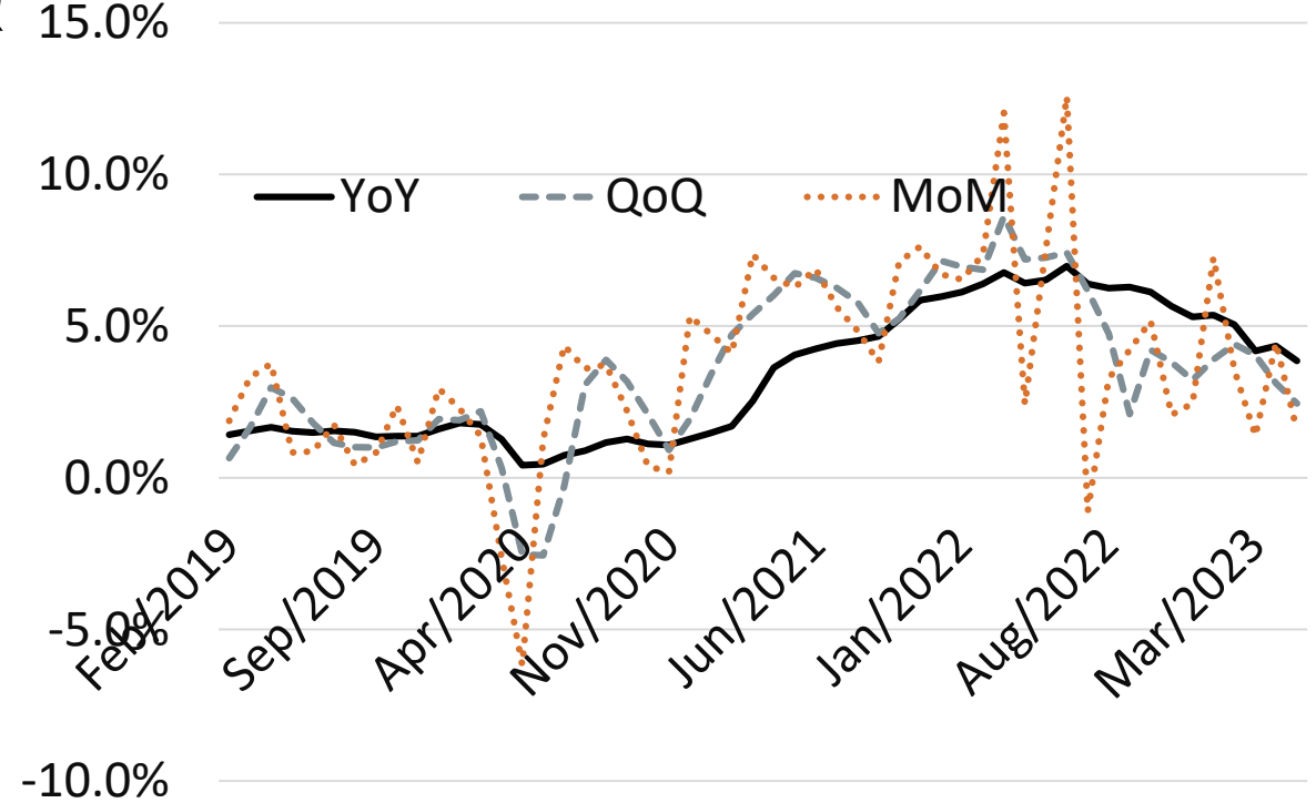
אינפלציה במונחים שנתיים, PCE
